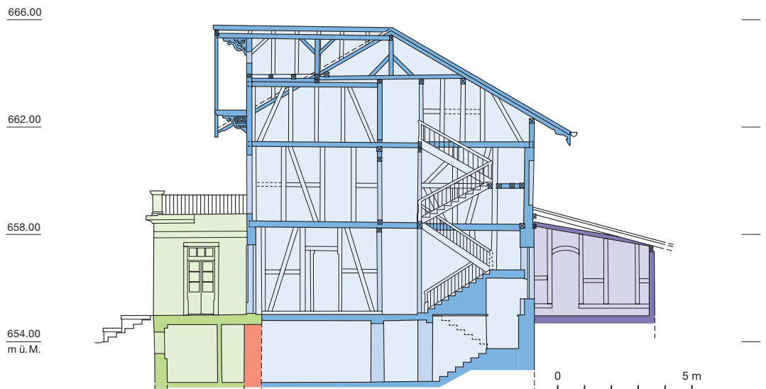
Abb. 4: Blumenstein, Badstrasse 37. Der Querschnitt durch das Gebäude zeigt das stockwerkweise abgebundene Tragwerk mit dem Treppenhaus (blau) und die teilweise geschlossene Veranda mit den darunterliegenden Badezimmern (grün), der nördliche Anbau (violett) erfolgte später. M. 1:200.
